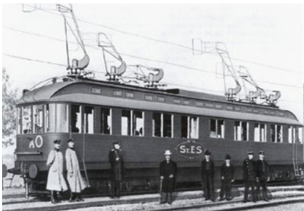
Bild 1: Drehstromversuchstriebwagen
