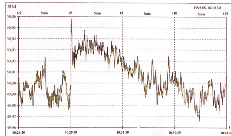
Bild 13: Probebetrieb CENTREL
