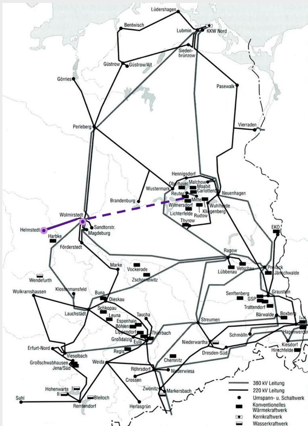
380-kV-Leitung Helmstedt–Wolmirstedt
